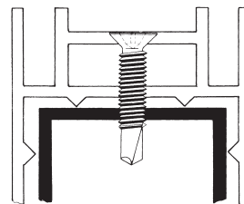
Typ FDM 1 - FDM 2 F
