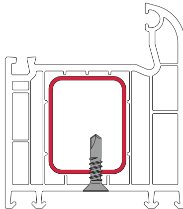
Schraubentyp 2
