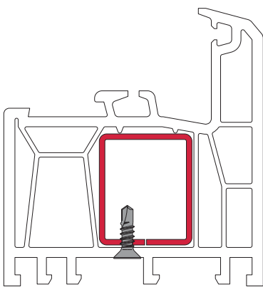
Schraubentyp 1
